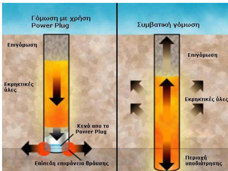
Βασική αρχή λειτουργίας της τάπας power plug
